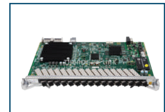
ZTE GFBT C+ D2
